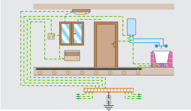
Liaison équipotentielle locale de la salle d'eau
